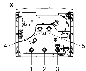
Vue de dessous CGB-2K
