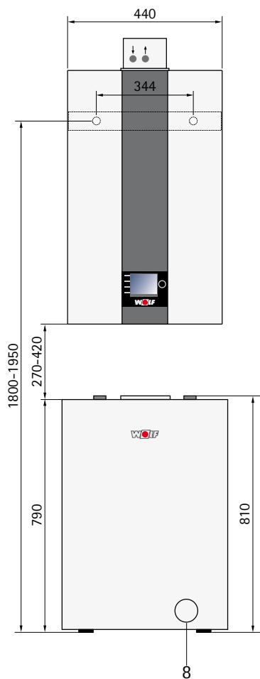
Vue de face CSW-120
