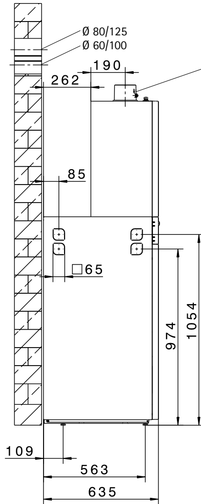
Vue de coté CGS-2R
