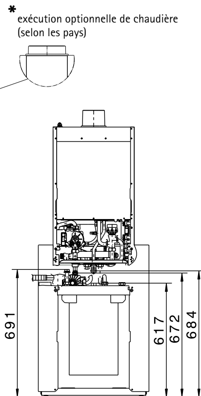
Vue de dos CGS-2L
