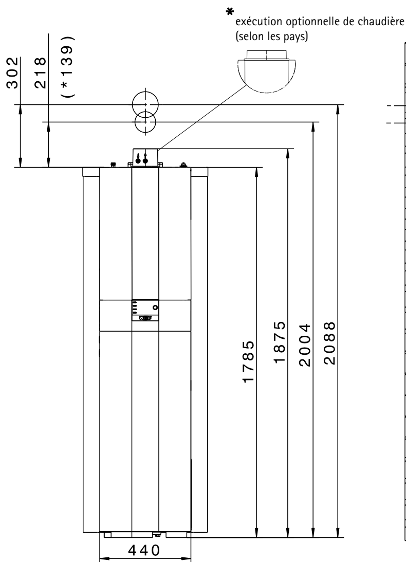
Vue de face CSZ-2R
