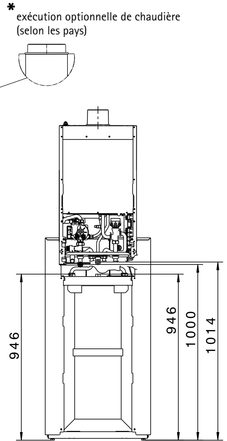
Vue de dos CGS-2R
